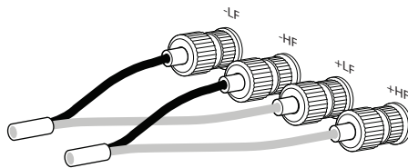
Connexion bi-câblée
